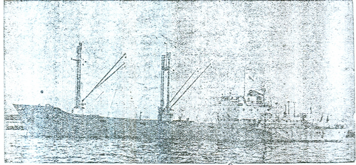
Eslera total, 73,55 metros. Manga, 11,60. Puntal cubierta superior, 6,80. Pantal cubierta principal, 4,55. Altura entrepuente, 2,25. Calado, 4,20. Capacidad de carga, porte bruto, 1.190 toneladas. Desplazamiento, 2.030 ton.
