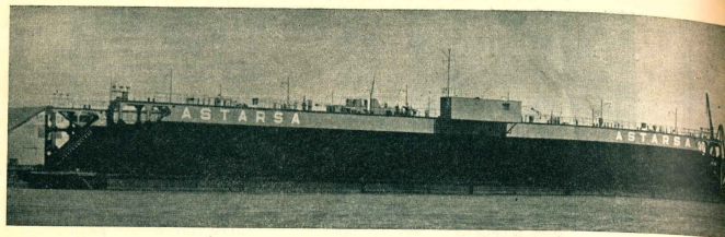
Dique Flotante ASTARSA. Construcción Nº 95. — Construcción efectuada en grados por secciones y unidas la misma a flote. Posee las siguientes características: 108,20 mts. de eslora, 24,20 de manga y 10,40 de puntal con una capacidad portante de 2.800 Tm., 5 pontones y 2 cojines laterales en los cuales están instaladas sus maquinarias y taller de mantenimiento. Construido durante los años 1955/56 para el M. T. N.
