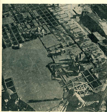
Plato de soldadura para grandes trozos.
